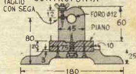
CONTROPUNTA
