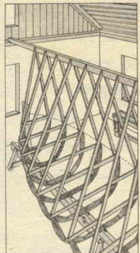
IMPOSTAZIONE DELLA CHIGLIA E DISTRIBUZIONE DELLE SESTE
